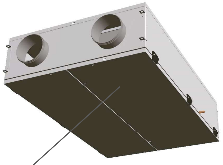
Pannello apribile (anta con cerniere) per accesso ai filtri IRSAIR H 430 - 600
