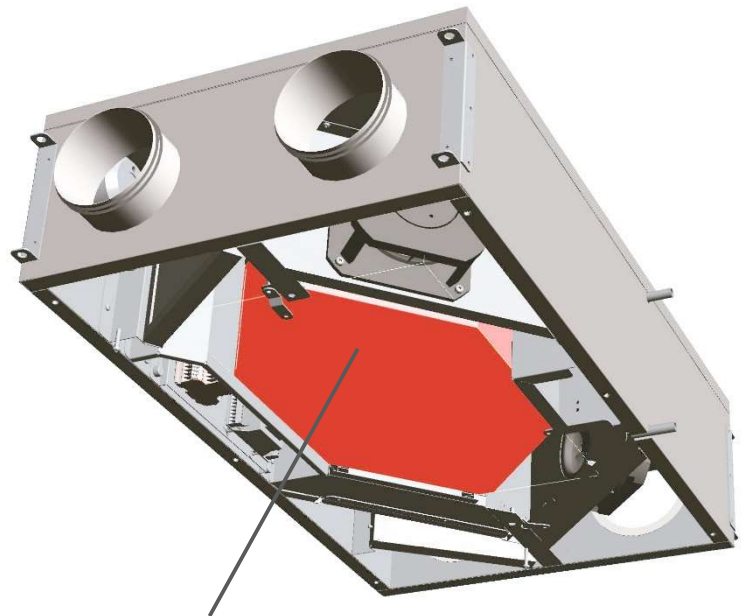
Scambiatore di calore IRSAIR H 150 - 220
