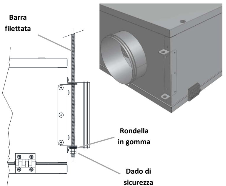
Montaggio a soffitto
