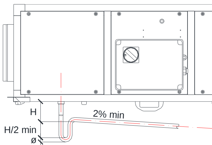
Allacciamento scarico condensa
