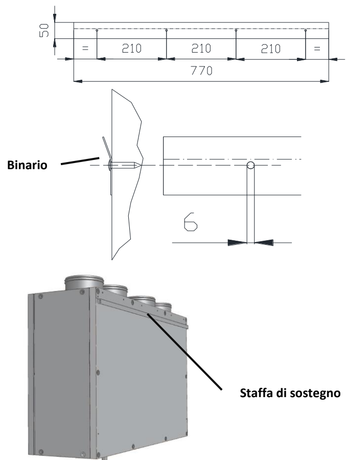
Montaggio a parete
