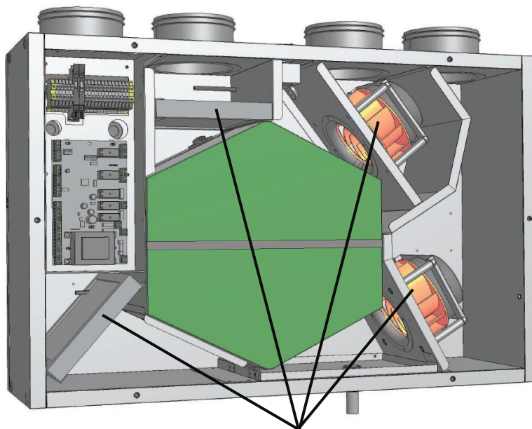
Filtri e ventilatori IRSAIR V 150
