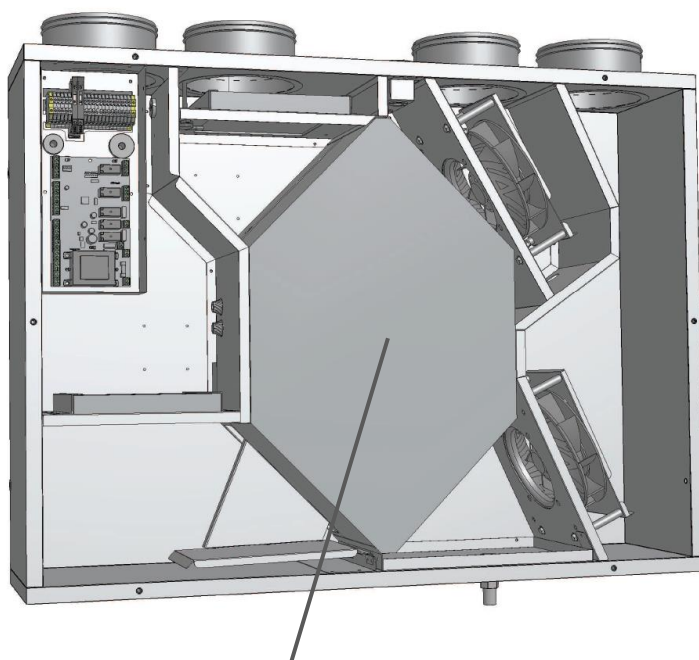
Scambiatore di calore IRSAIR H 350 - 500
