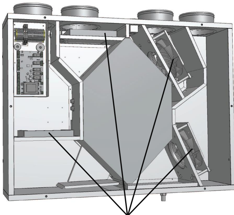
Filtri e ventilatori IRSAIR V220
