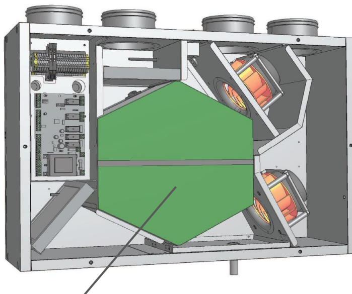
Scambiatore di calore IRSAIR V 150
