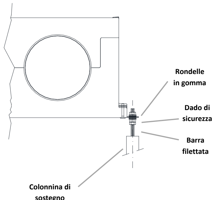
Montaggio a pavimento
