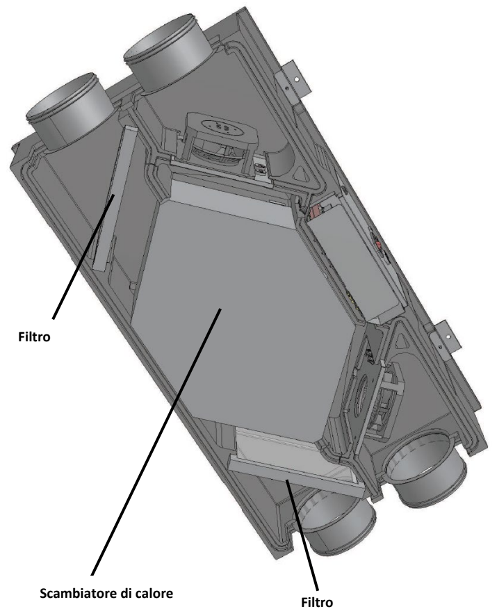
Estrazione scambiatore
