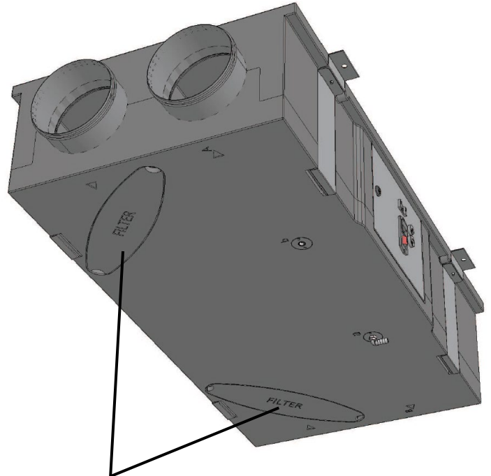
Coperchi di accesso ai filtri IRSAIR H 150 P – 220 P
